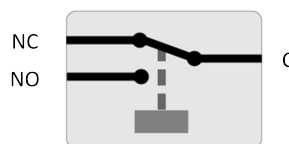
Relaiskonfiguration (nicht angezogen).
