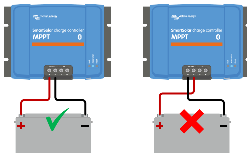
Beispiele für richtige und falsche (vertauschte) Batteriepolareität
