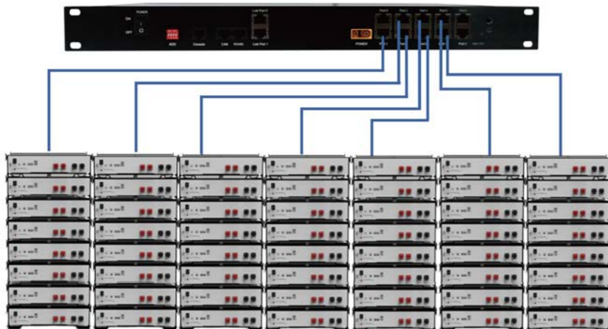
Jede Gruppe unterstützt maximal 8 Stück E-BOX-4850 oder E-BOX-48100 parallel
